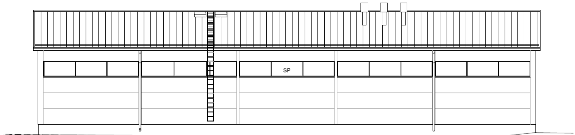
JULKISIVU ETELÄÄN
